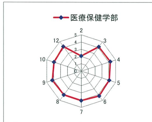
評価点数
